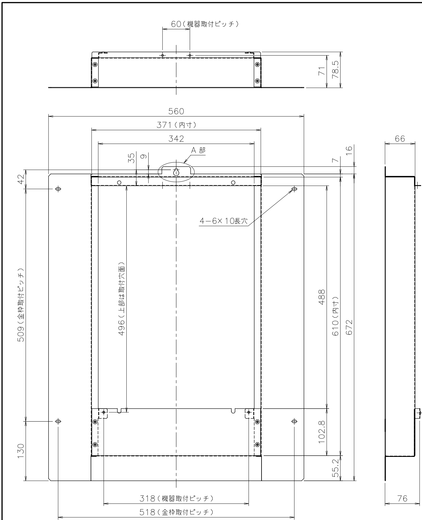
■ 取付参考図
