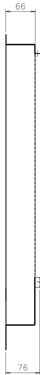
■ A部詳細 (尺度 1/1)
