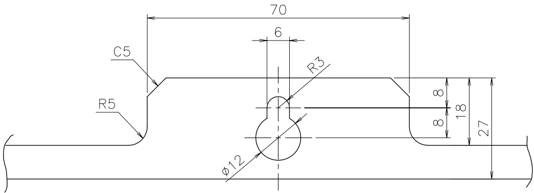
■ A部詳細（尺度1／1）
