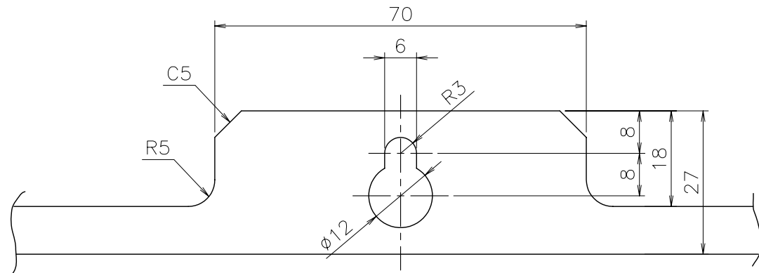
■A部詳細（尺度1/1）
