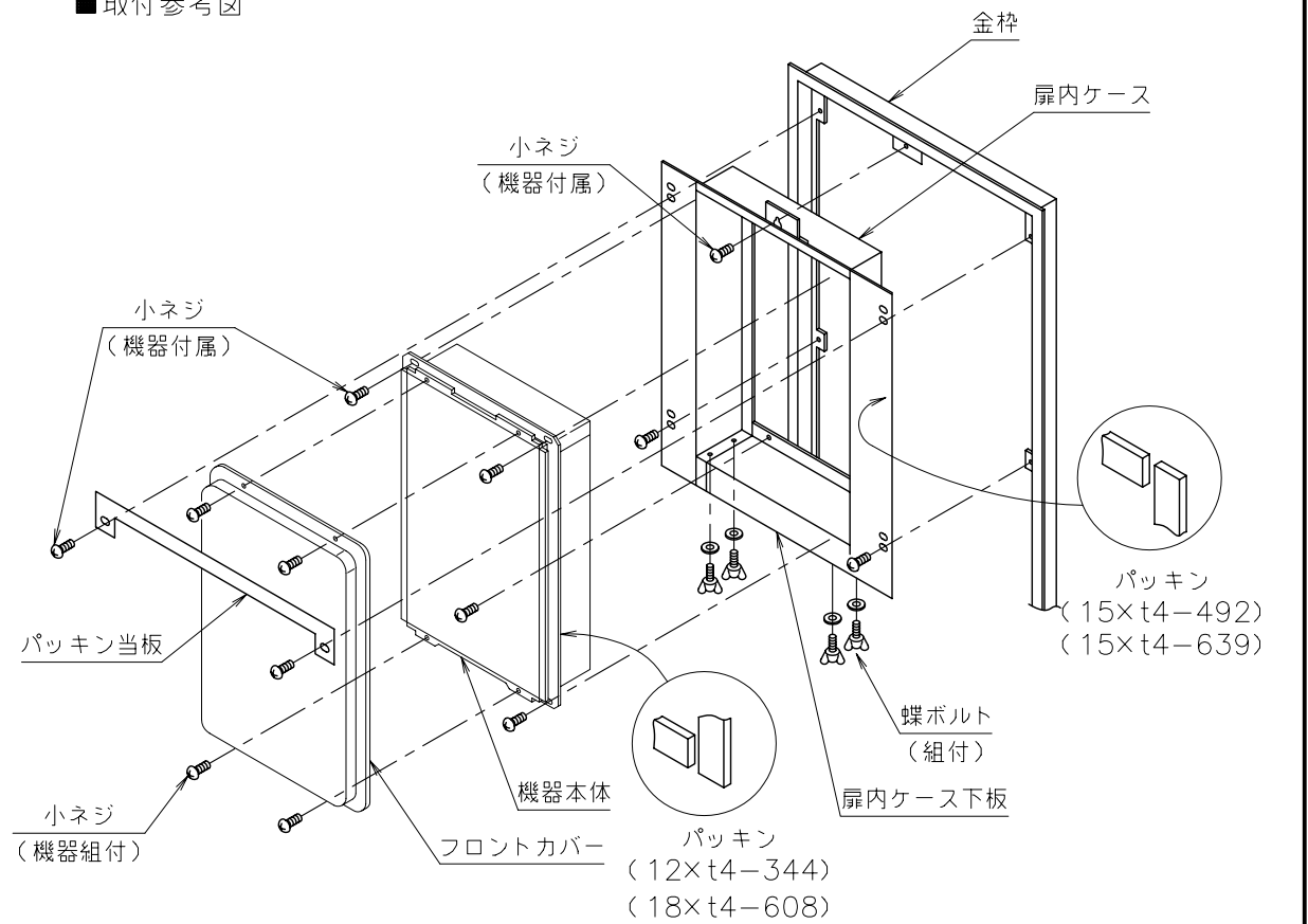
■取付参考図
