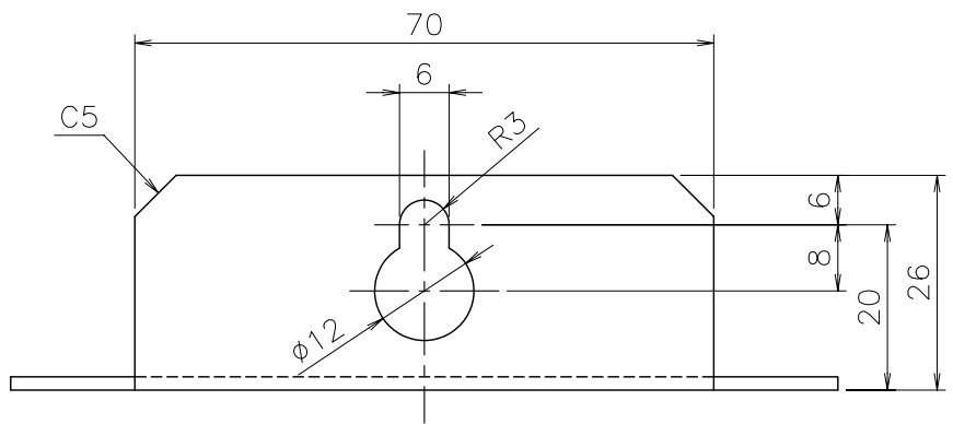
■A部詳細 (尺度 1/1)
