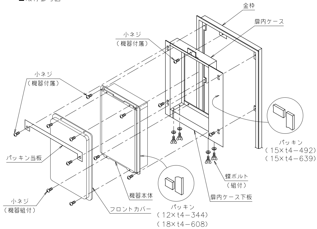
■取付参考図
