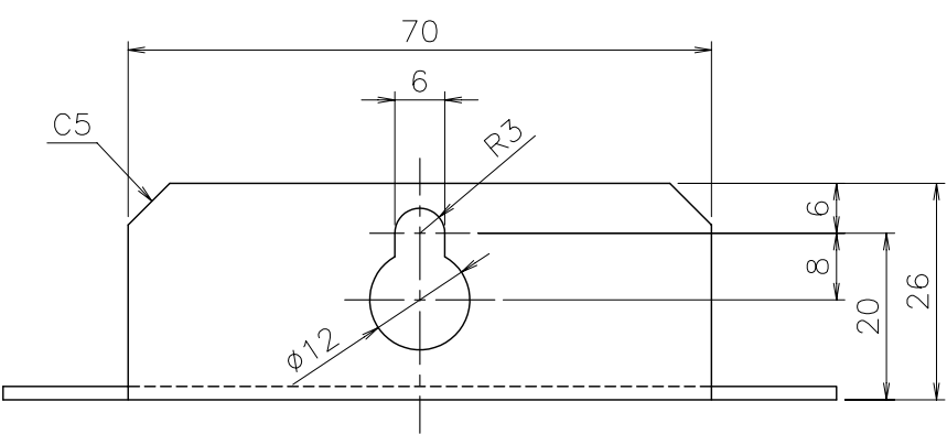
■A部詳細 (尺度 1/1)
