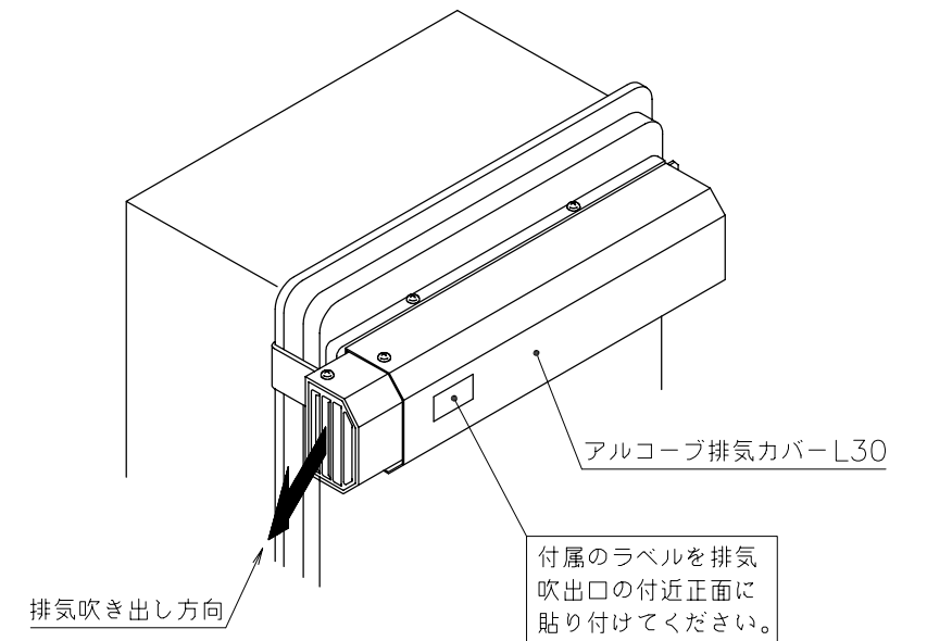
取付完成図（概略）
