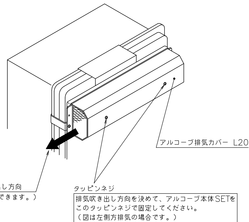
取付完成図（概略）
