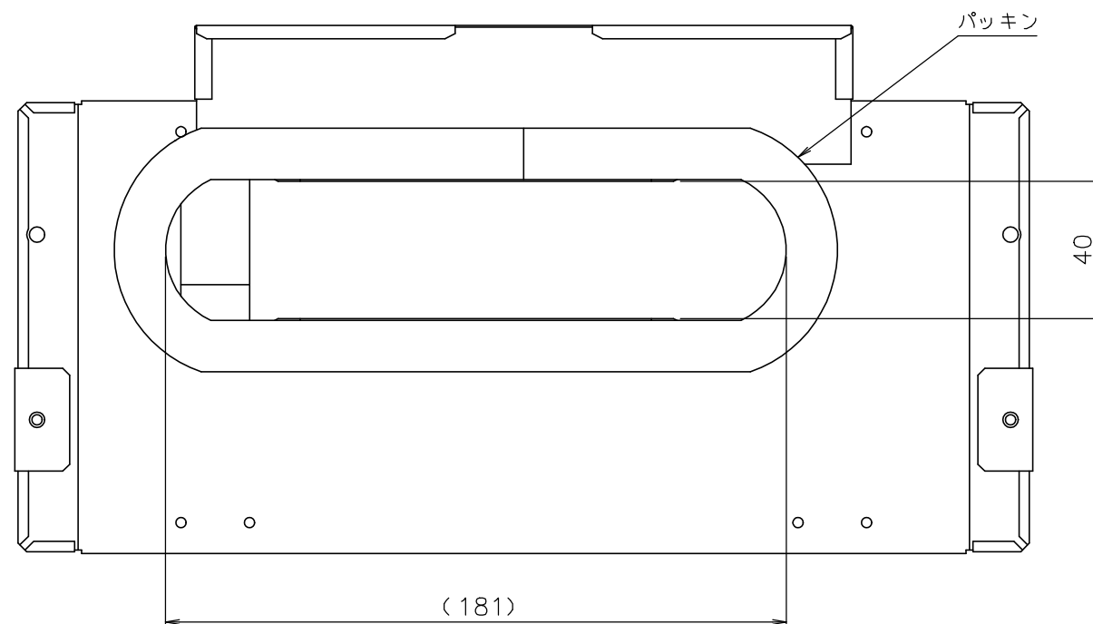
矢視A（排気カバー裏面）
