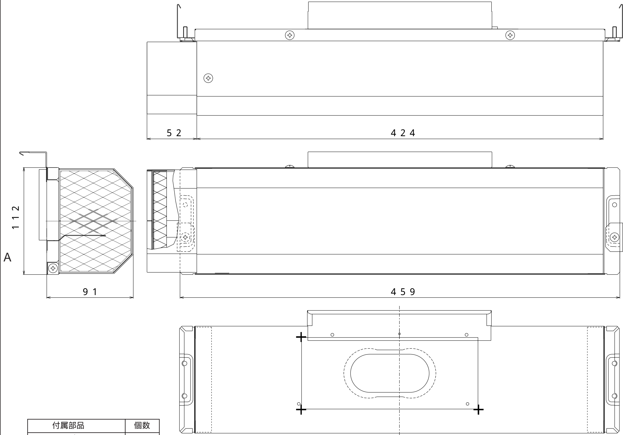
矢視A（排気カバー裏面）
