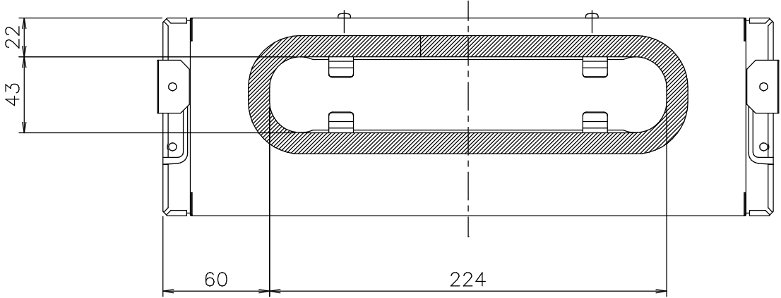
矢視A（排気カバー裏面）
