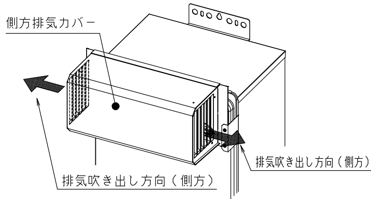
取付完了図（概略）
