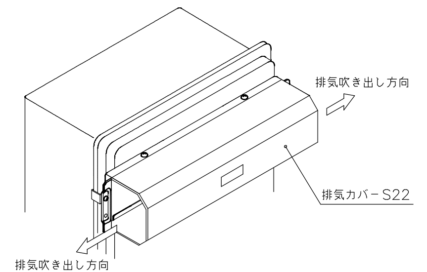
取付完了図（概略）
