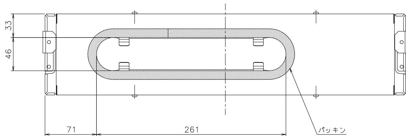
矢視A（排気カバー裏面）
