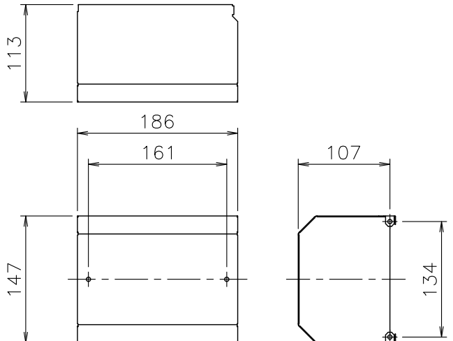
■化粧カバー寸法図
