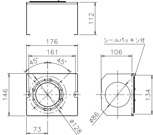
■化粧カバー寸法図
