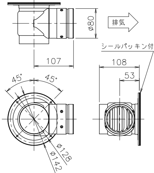
■ 固定金具寸法図
