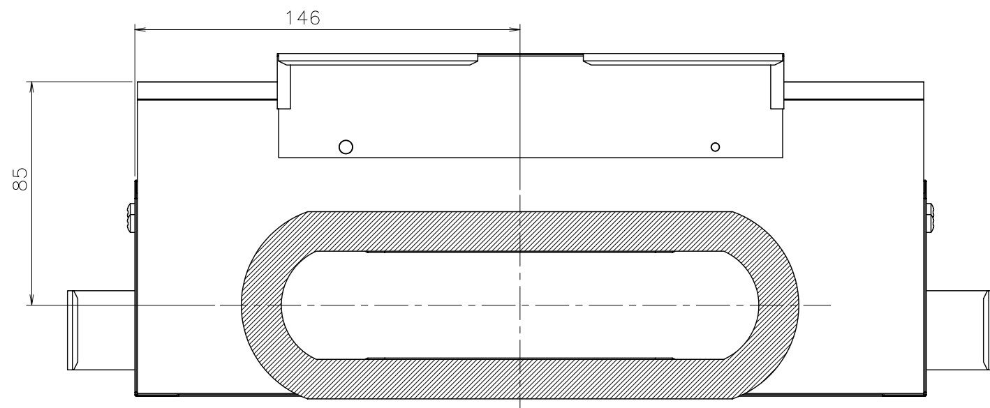
矢視A
