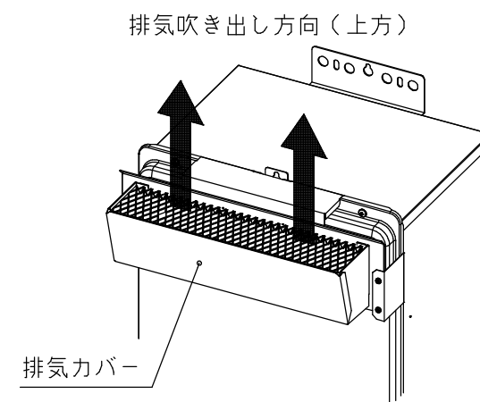
取付完了図 (概略)
