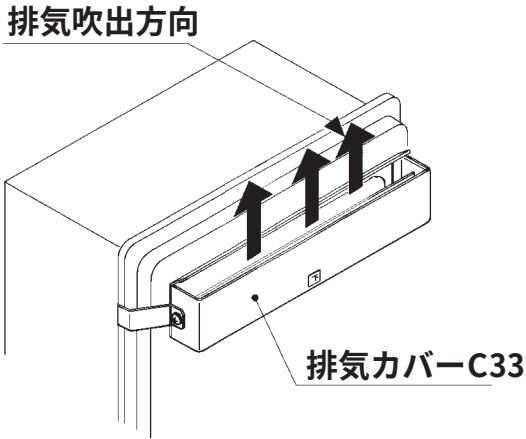
取付完成図（概略）
