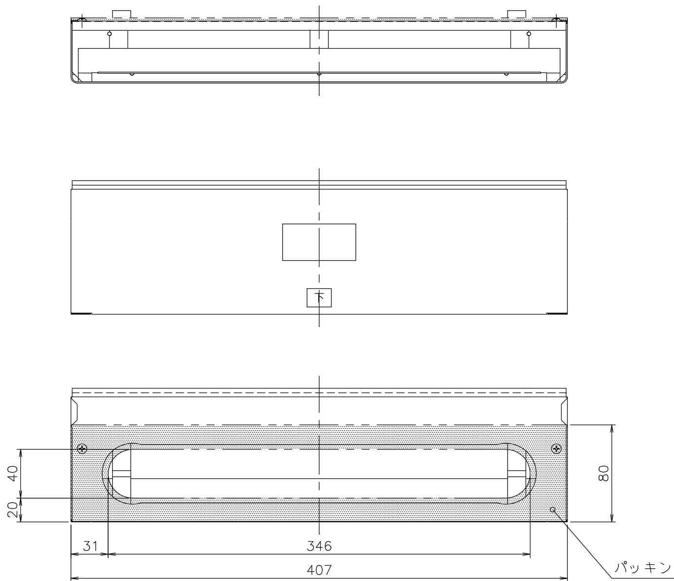
矢視A（排気カバー裏面）
