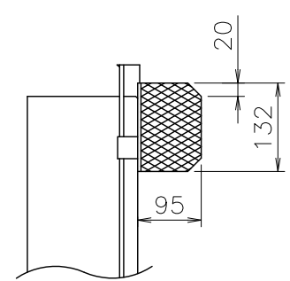
■アルコーブ取付図
