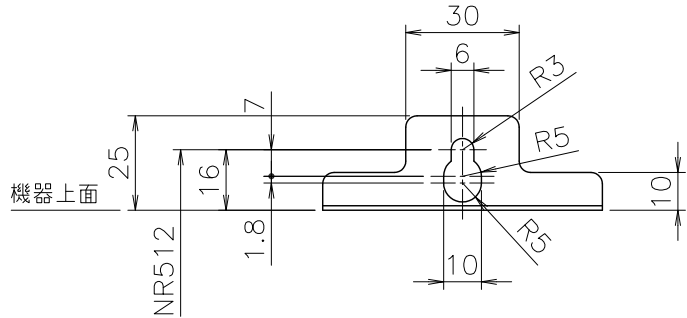
■A部詳細図（尺度1／2）
