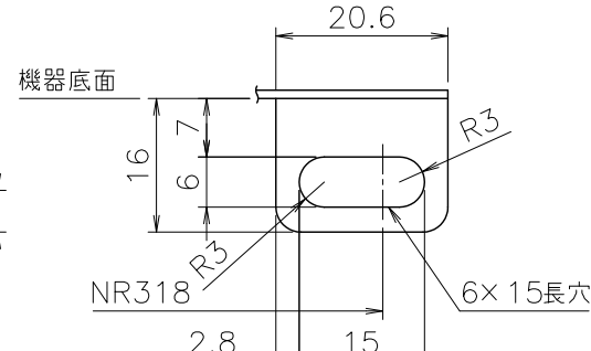
■B部詳細図（尺度1／1）
