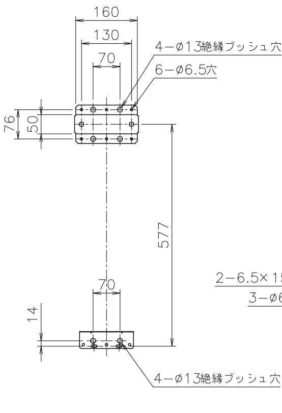
参考 （壁掛金具 AGV使用時）
