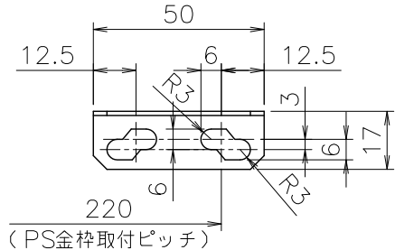
■B部詳細図（尺度1／2）
