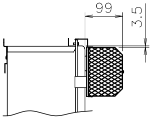
■アルコーブ取付図
