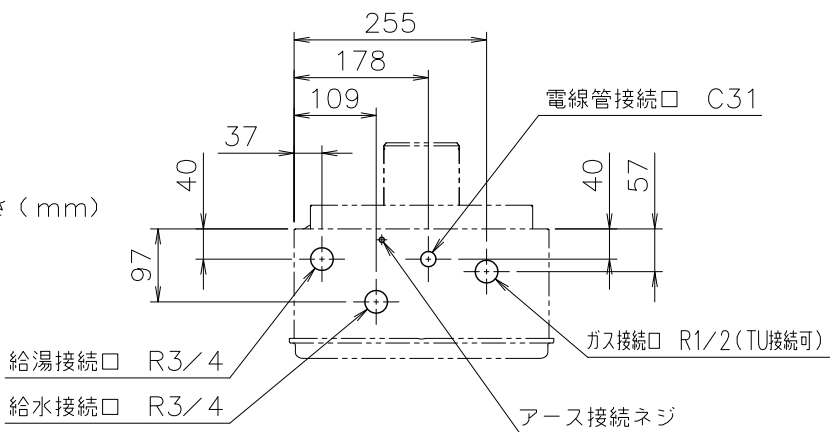
（機器上方よりの透視図）
