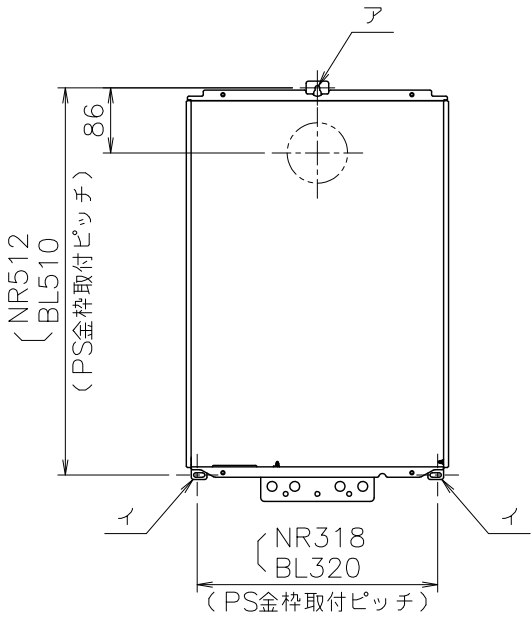
（フロントカバーを外した状態）
