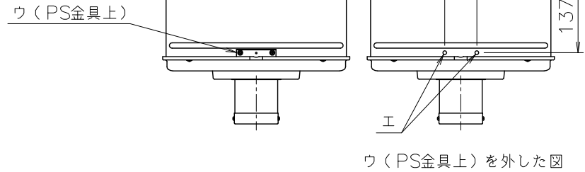
ウ（PS金具上）を外した図
