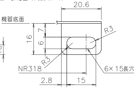
■イ詳細図（尺度1／1）
