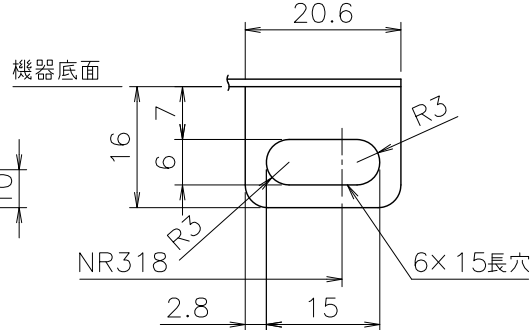
■イ詳細図（尺度1／1）
