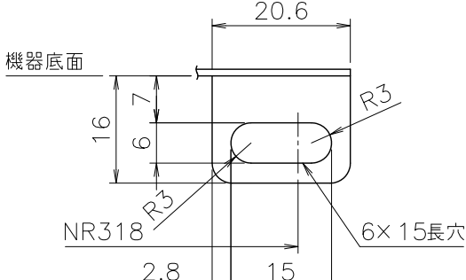
■イ部詳細図（尺度1／1）
