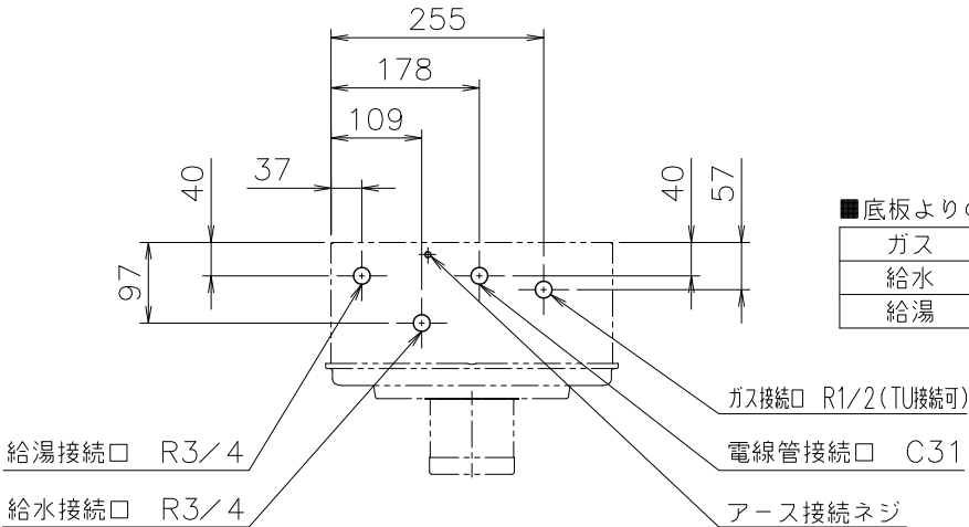
（機器上方よりの透視図）
