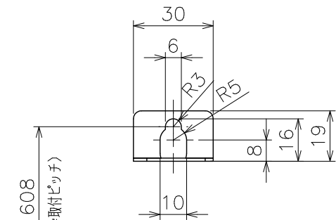
■ア部詳細 (S=1/2)
