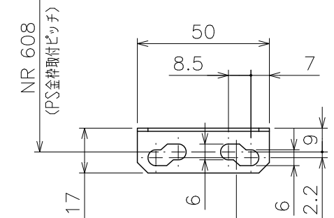
■イ部詳細 (S=1/2)
