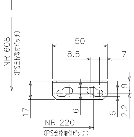
■イ部詳細 (S=1/2)
