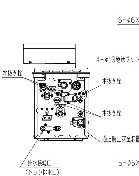
6-φ6×10長穴
