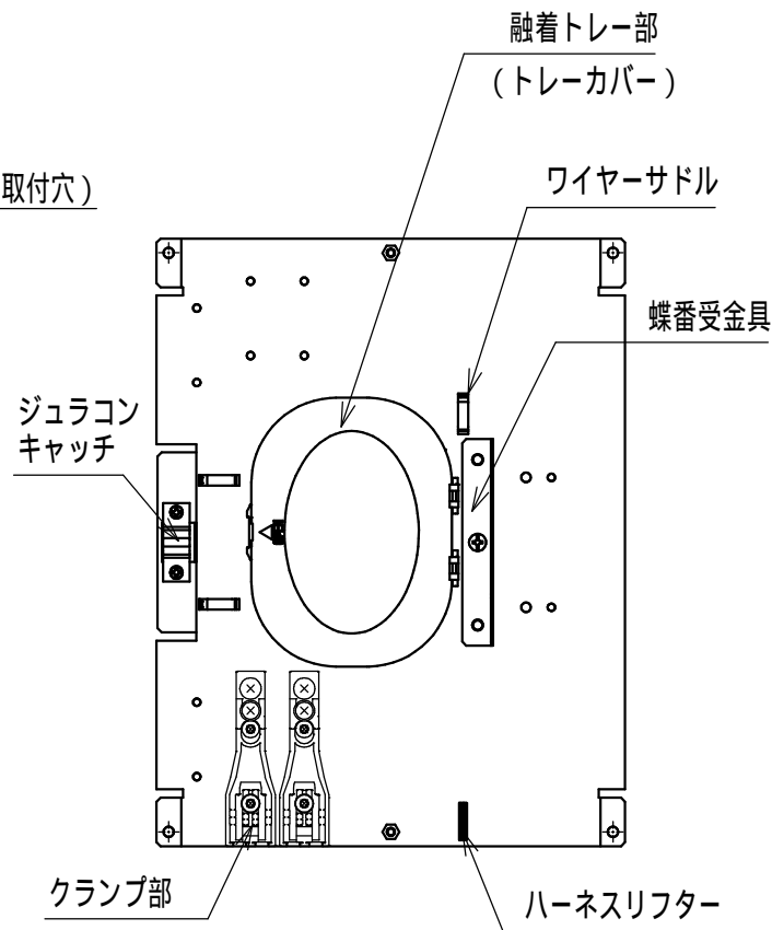
内部詳細図
