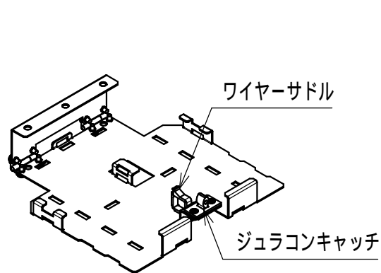
メディコン取付ベース
