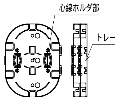
融着トレー部 (1:4)
