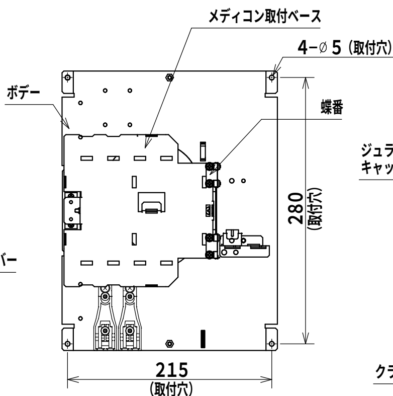
内部詳細図
