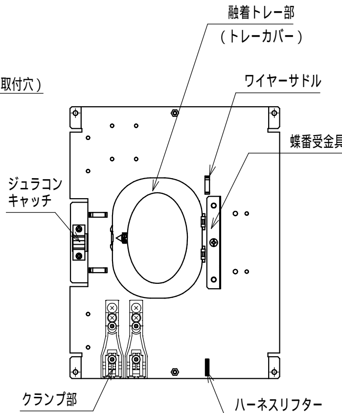
内部詳細図
