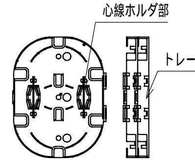
融着トレ-部 (1:4)
