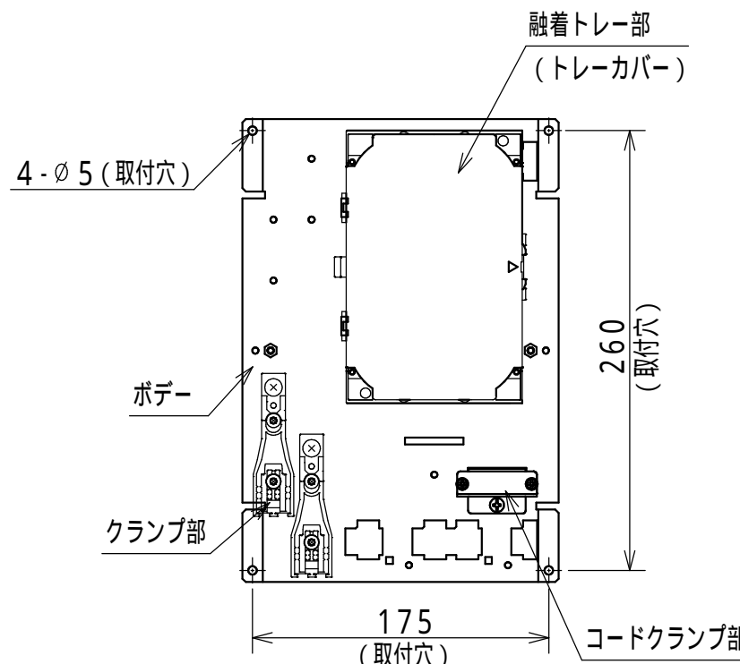
内部詳細図
