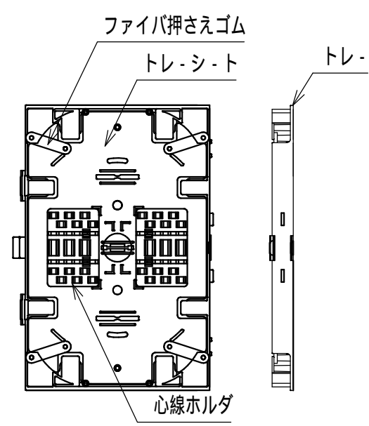
融着トレ-部 (1:3)
