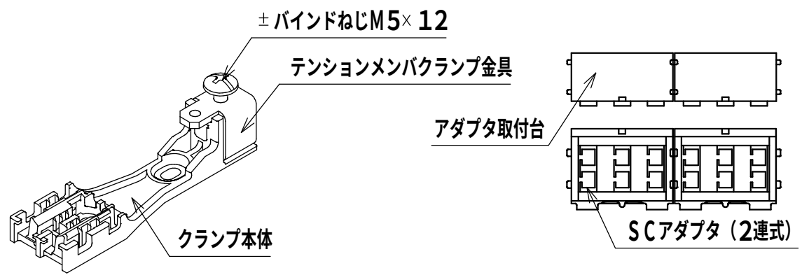
リール台 (1:3) 融着トレー部 (1:3) クランプ部 SCアダプタ部 (1:3)
