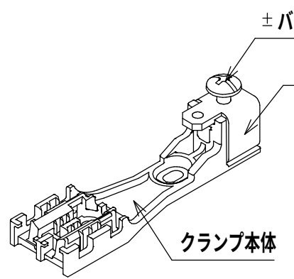
クランプ部
