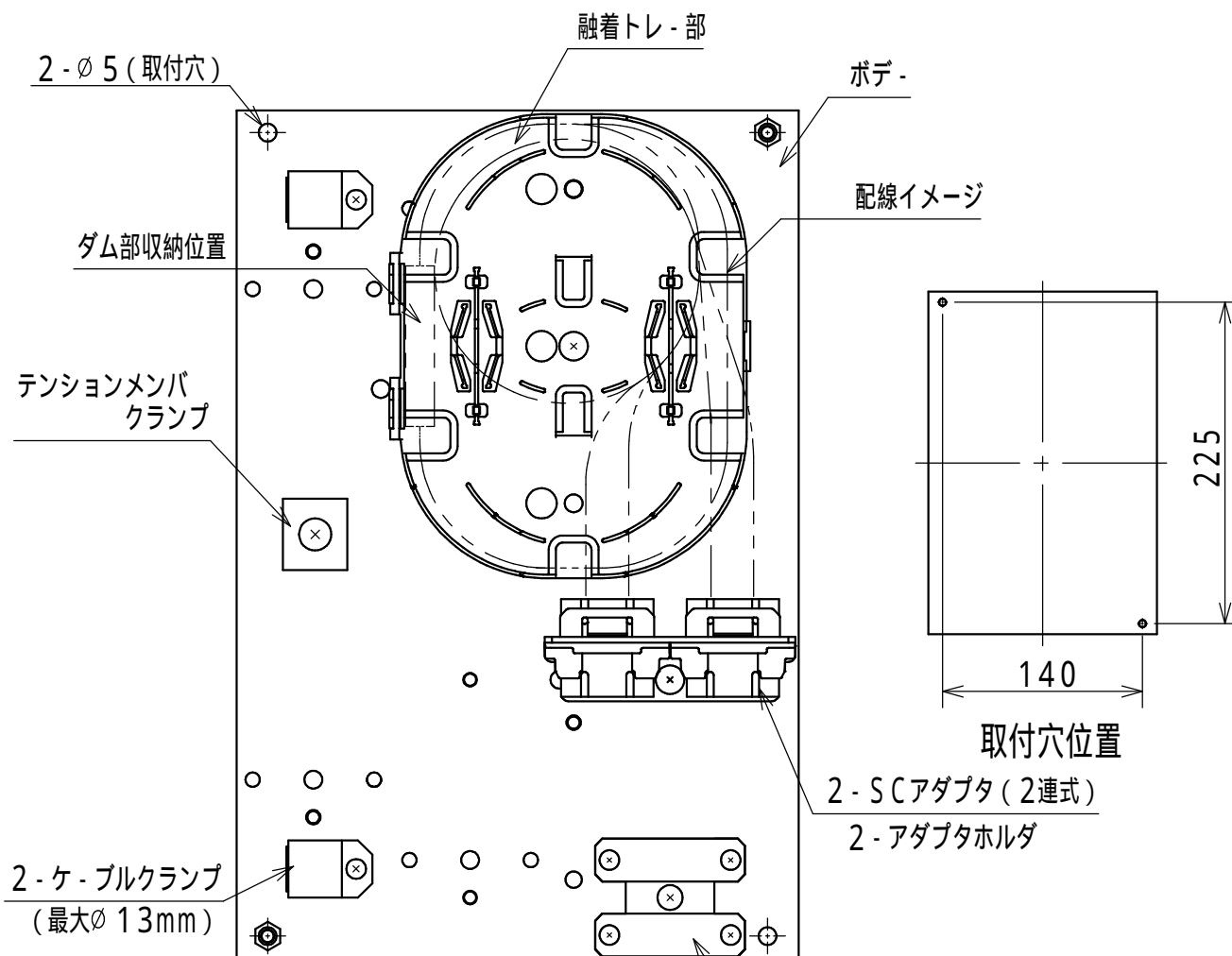
内部詳細図
