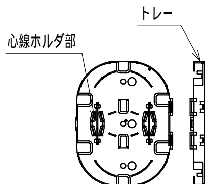
融着トレ部 (1:4)
