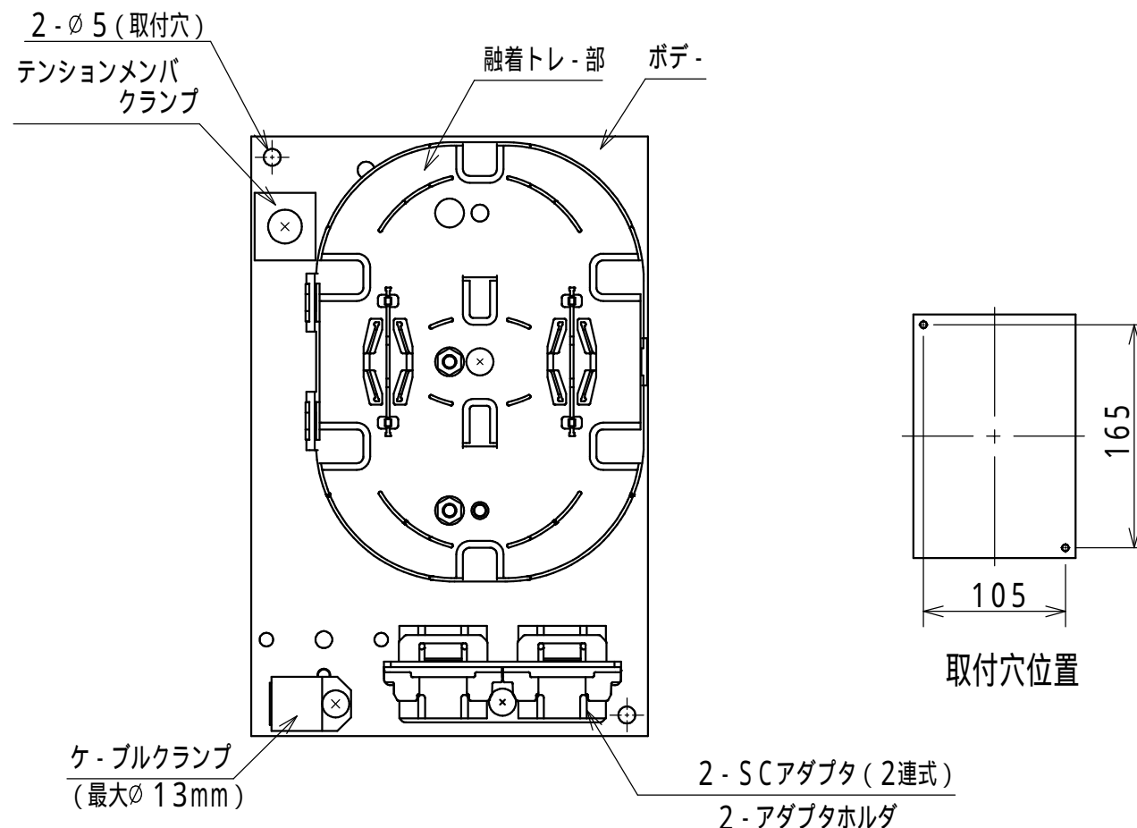
内部詳細図
