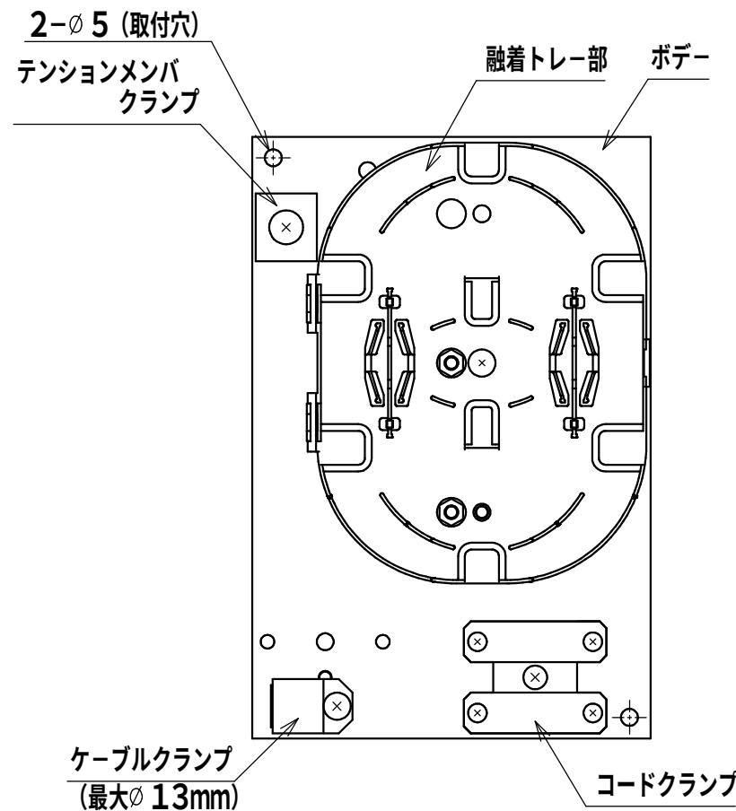
内部詳細図
