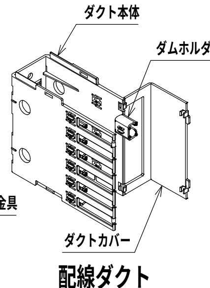
内部詳細図
