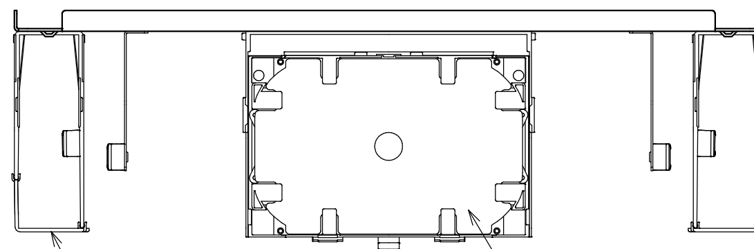
融着ユニット (1:3)
