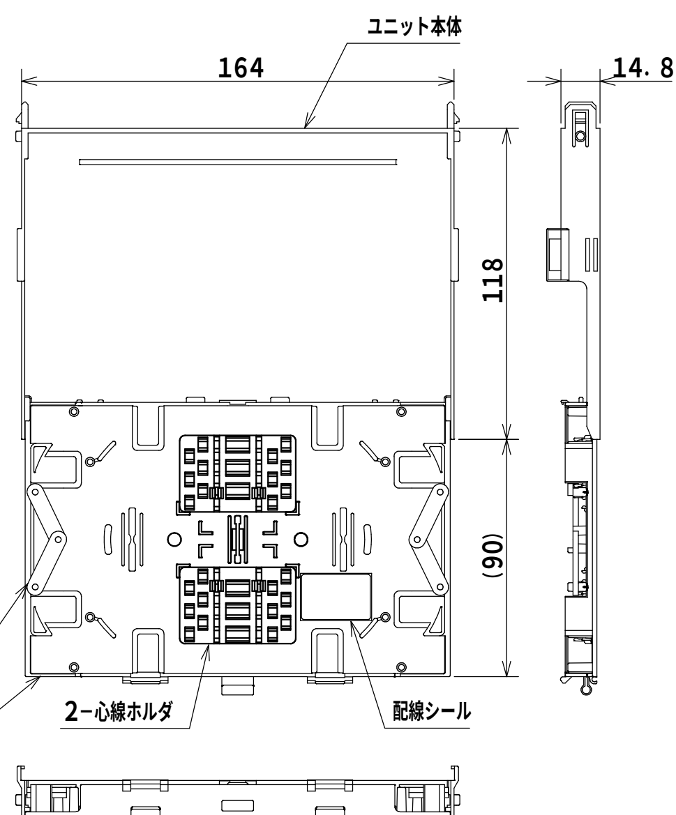
融着ユニット (1:3)
