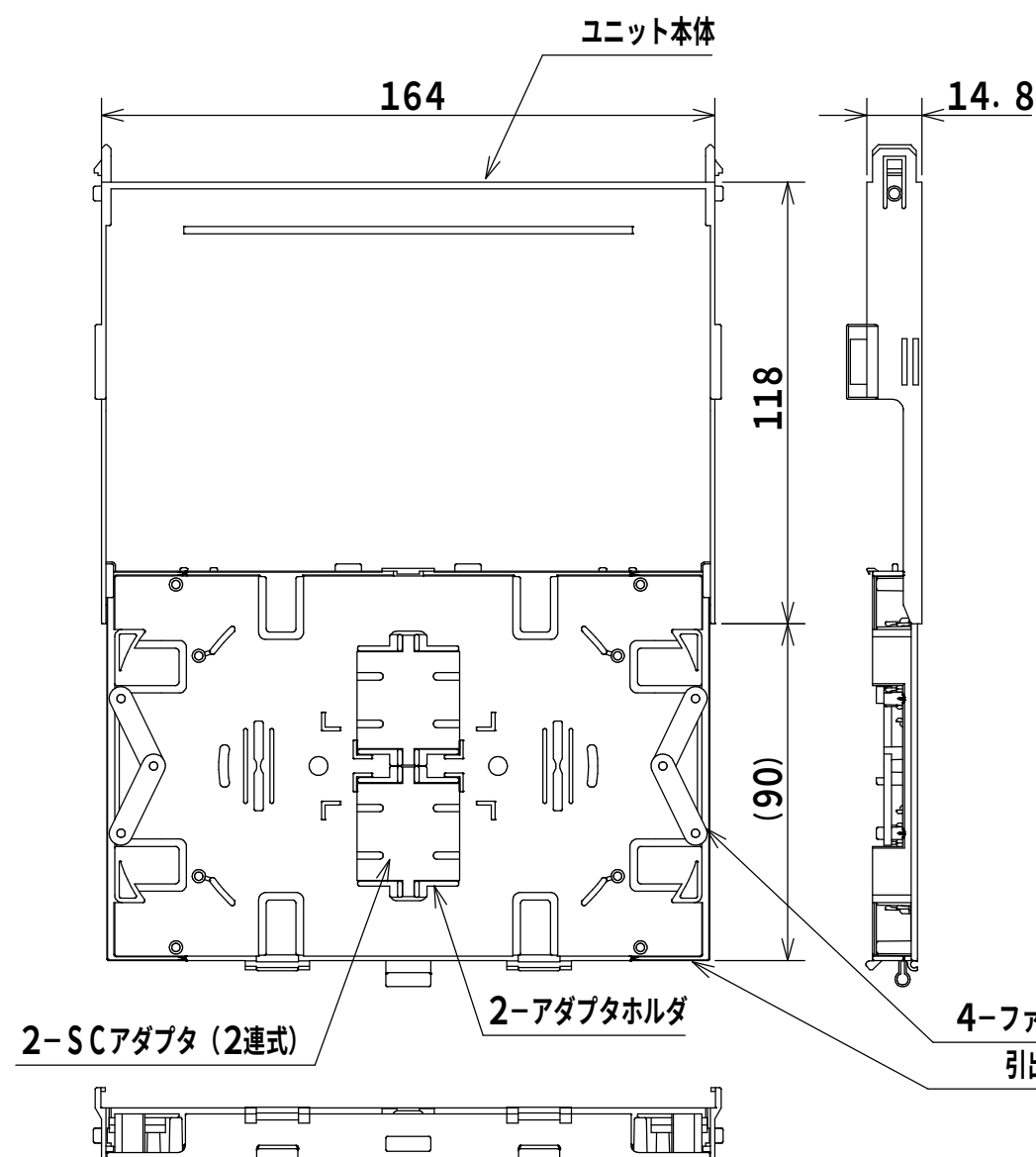
アダプタユニット (1:3)
