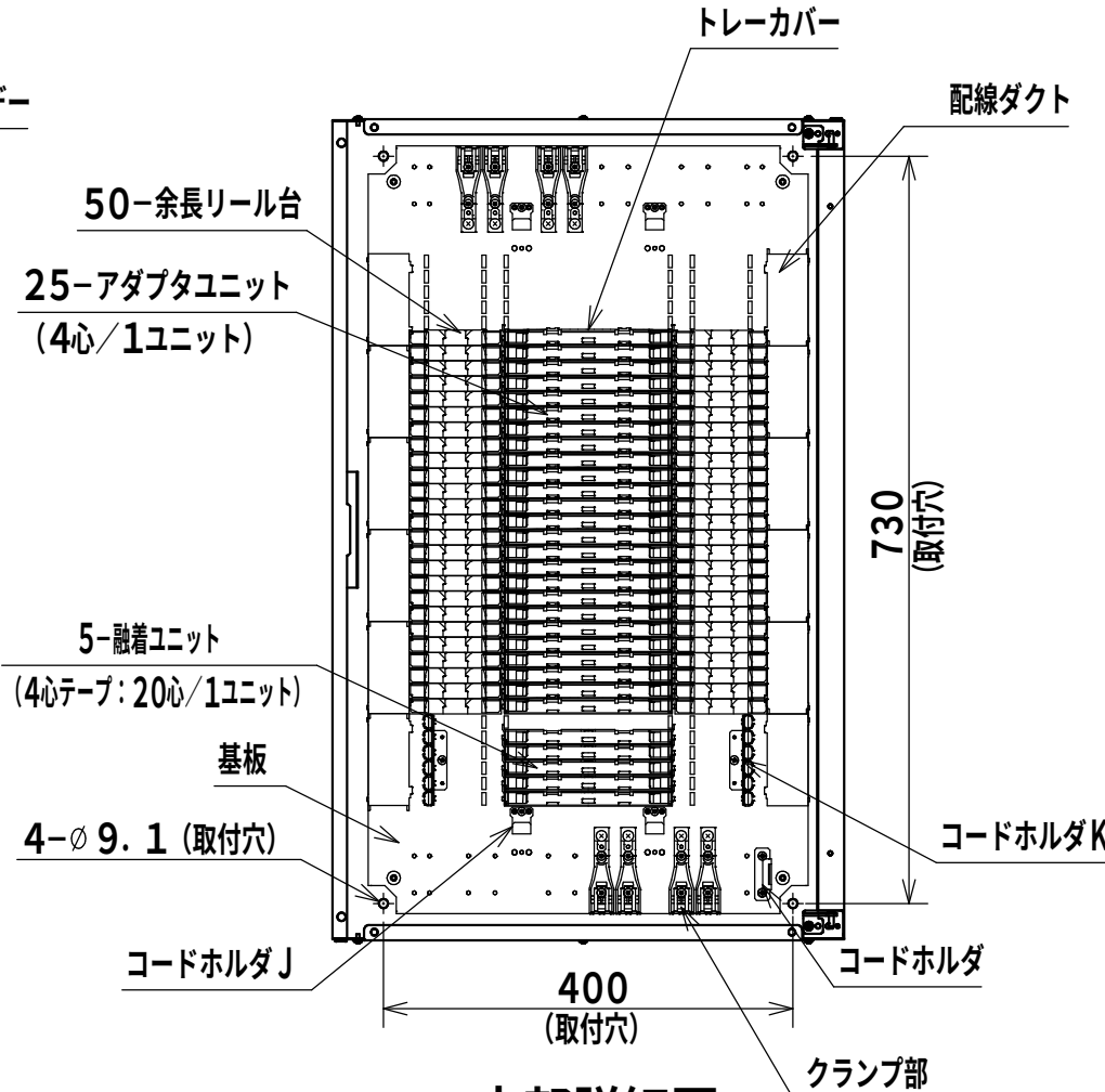
内部詳細図
