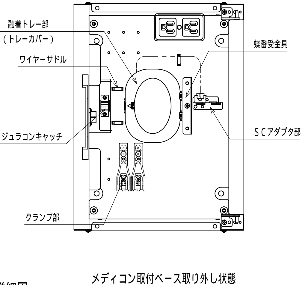
内部詳細図
