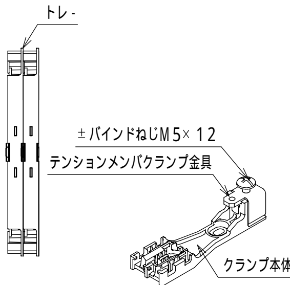
クランプ部
