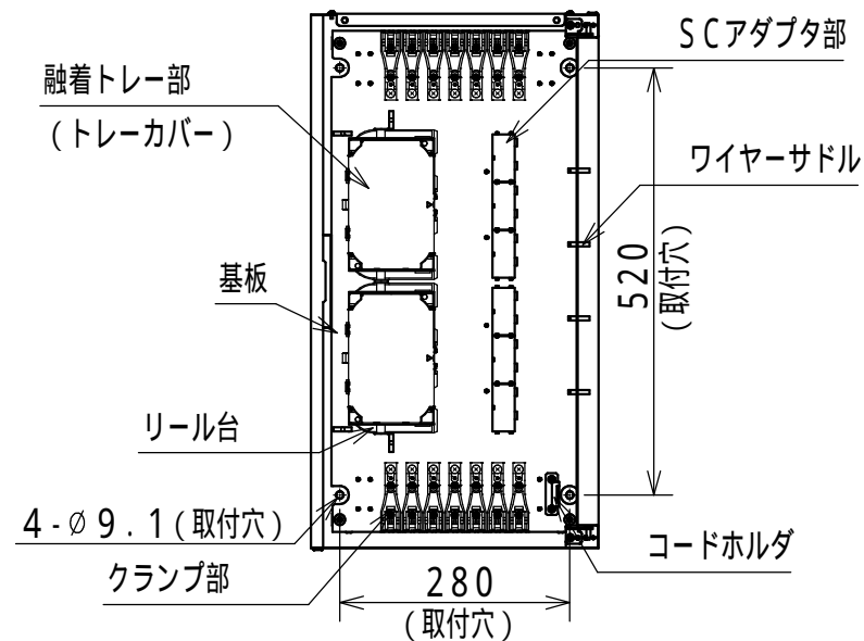
内部詳細図
