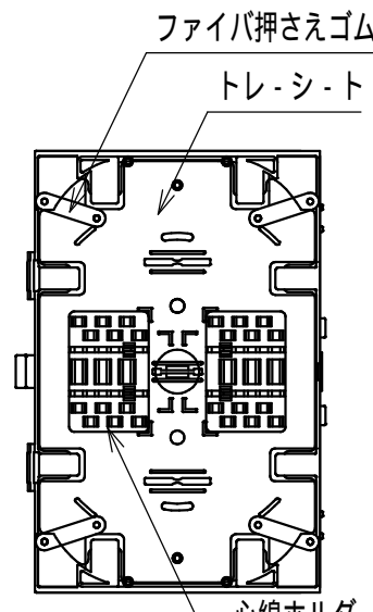
融着トレ-部 (1:3)
