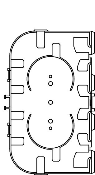
リール台 (1:3)
