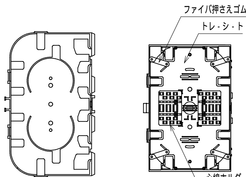
リール台 (1:3)
