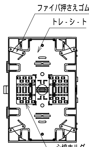
融着トレ-部 (1:3)
