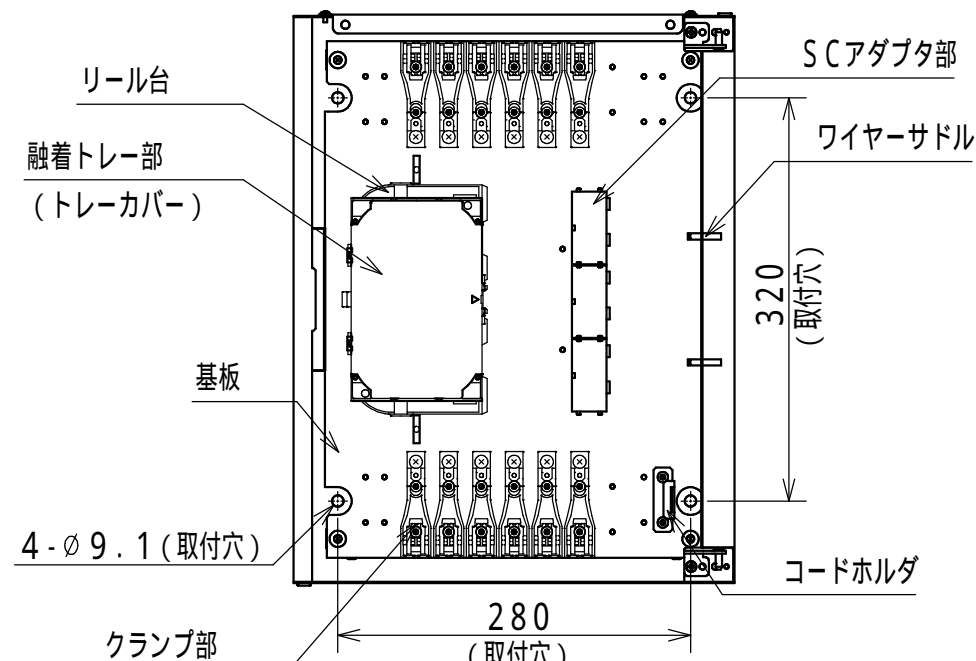
内部詳細図
