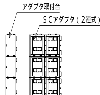
SCアダプタ部 (1:5)
