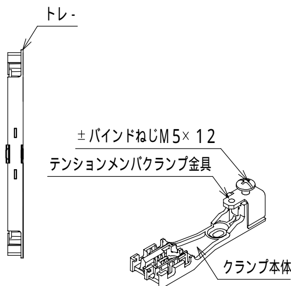
クランプ部
