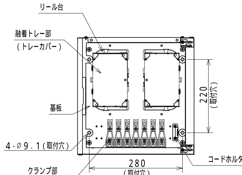
内部詳細図
