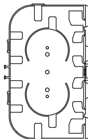
リール台 (1:3)
