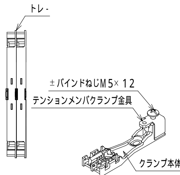
クランプ部
