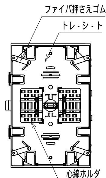
融着トレ-部 (1:3)
