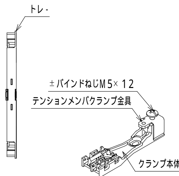
クランプ部
