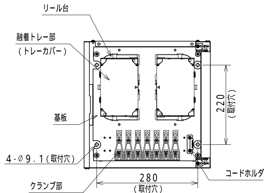
内部詳細図
