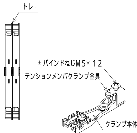
クランプ部
