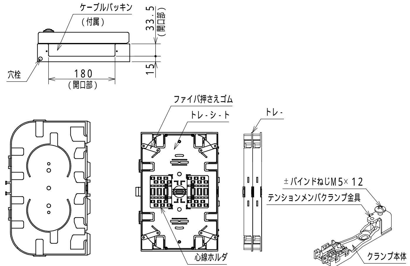
リール台 (1:3) 融着トレ-部 (1:3) クランプ部
