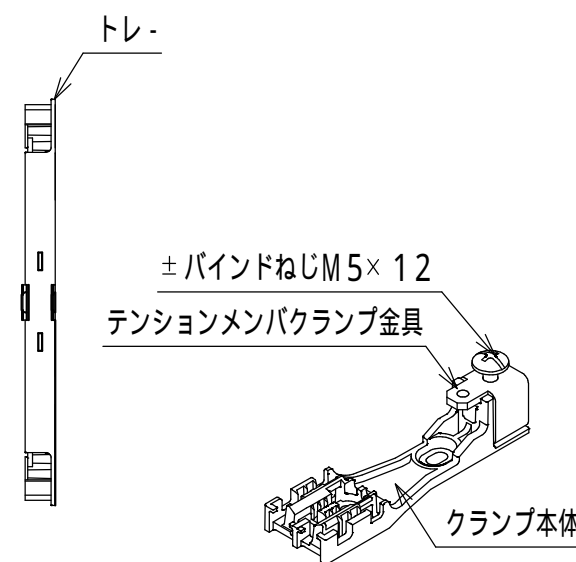
クランプ部
