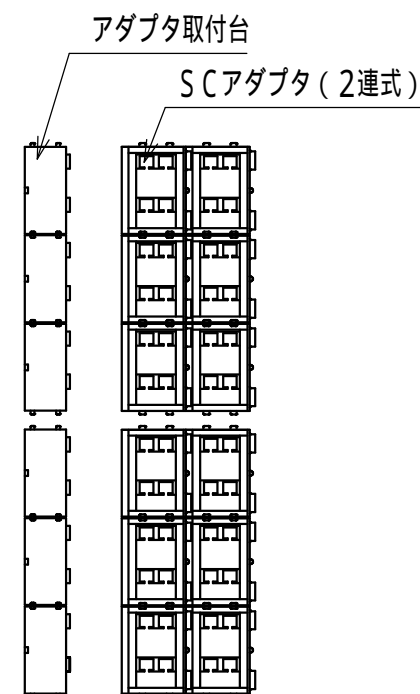
SCアダプタ部 (1:5)
