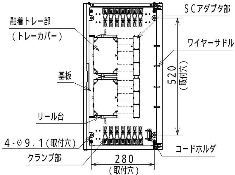
内部詳細図
