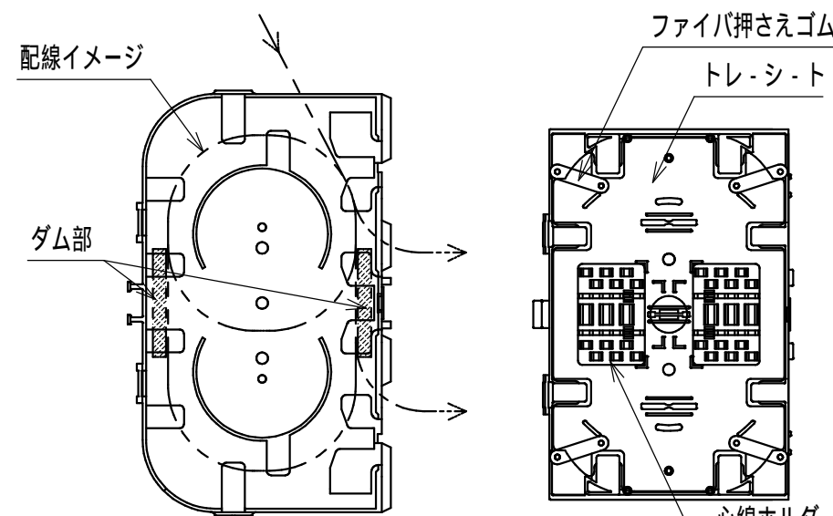
リール台 (1:3)
