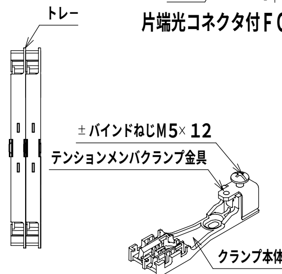
クランプ部
