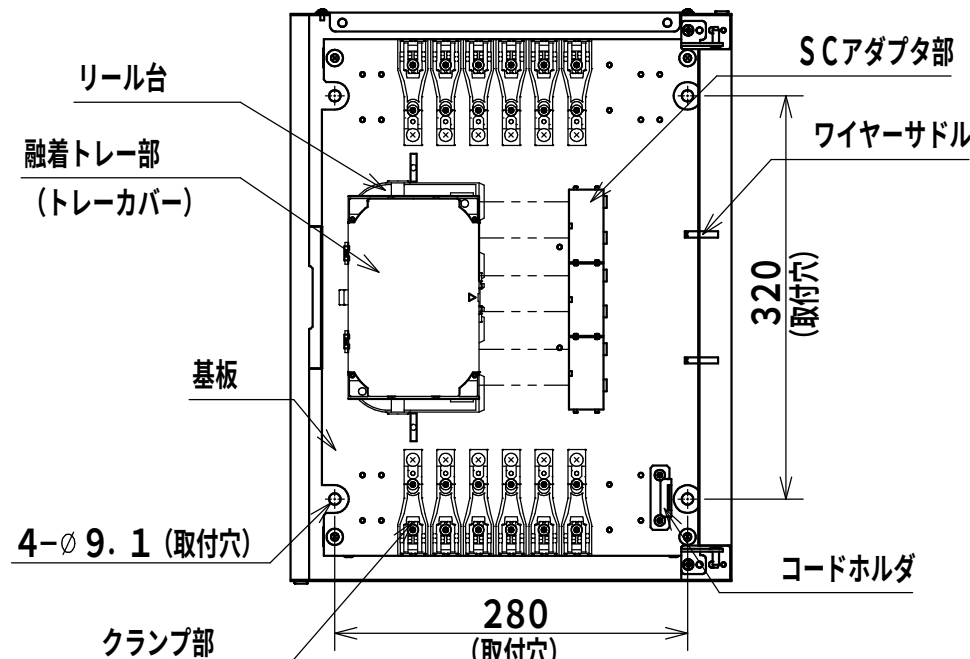
内部詳細図
