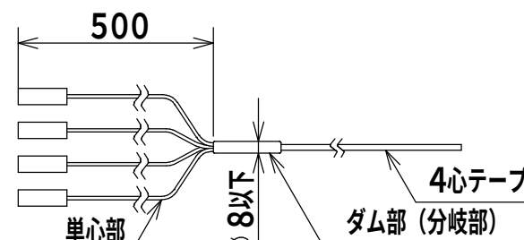
片端光コネクタ付FOコード推奨寸法
