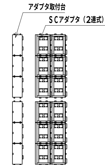
SCアダプタ部 (1:5)
