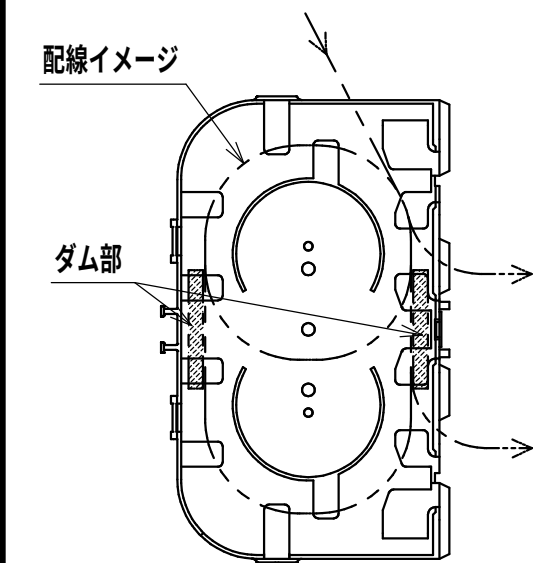
リール台 (1:3)
