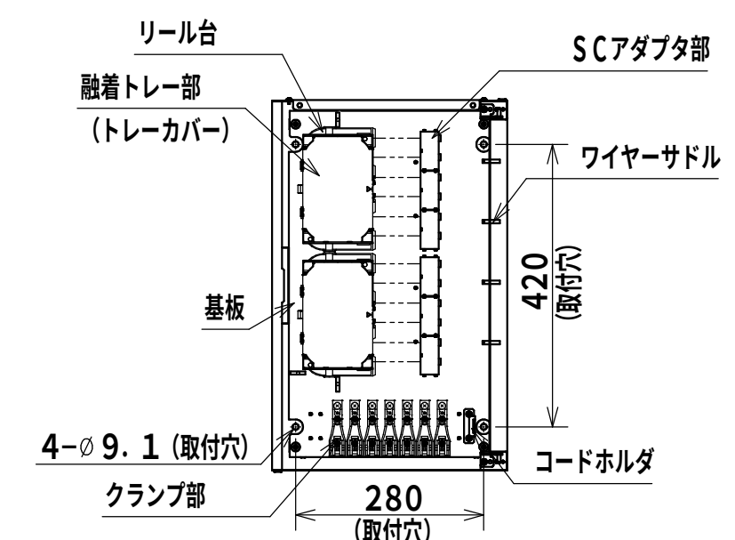
内部詳細図
