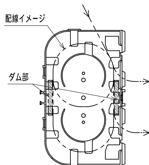
リール台 (1:3)
