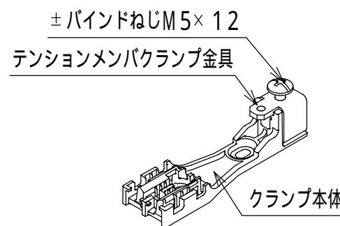
クランプ部
