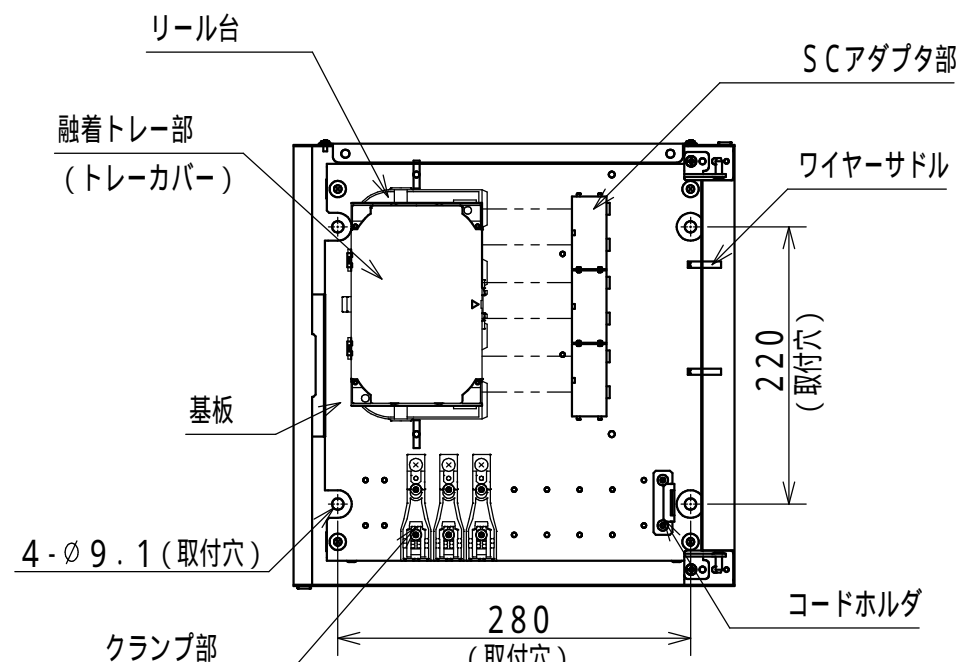
内部詳細図
