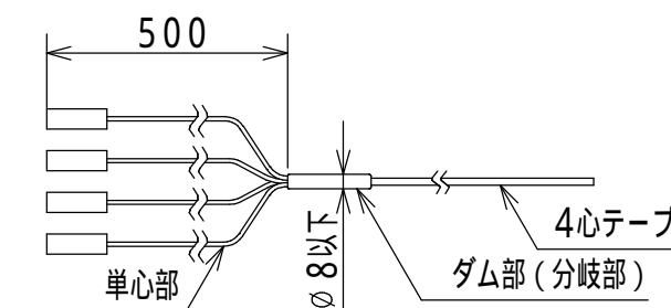
片端光コネクタ付F0コード推奨寸法
