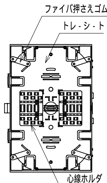
融着トレ-部 (1:3)
