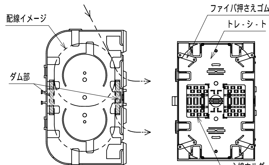
リール台 (1:3)
