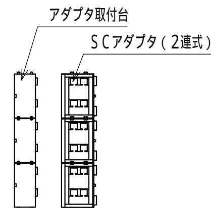
SCアダプタ部 (1:5)
